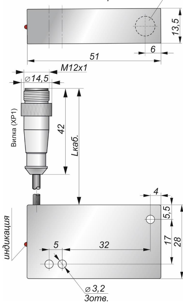
Габаритный чертеж
