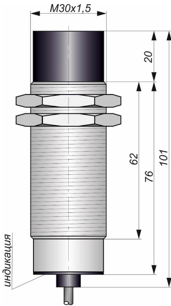
Габаритный чертеж
