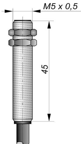
Габаритный чертеж
