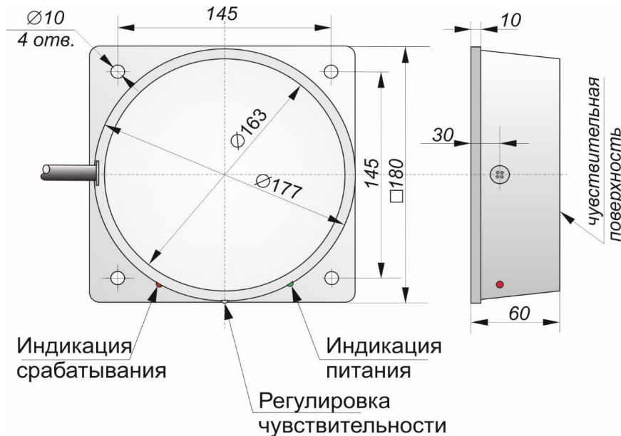
Габаритный чертеж
